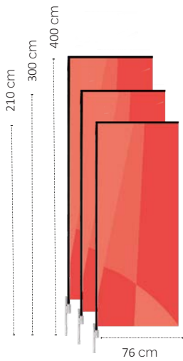
H Flag
