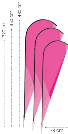
Tipa Flag
